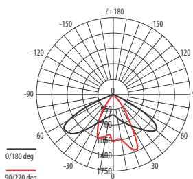
PSL 03 30W 5000K IP65
