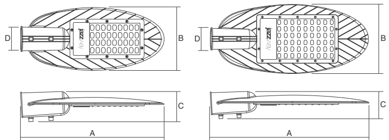
PSL 03 30W 5000K IP65
